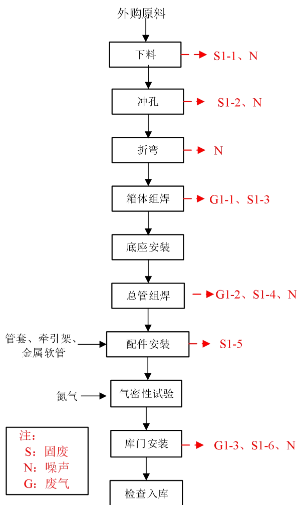
图 3-2 单冻机生产工艺流程图
