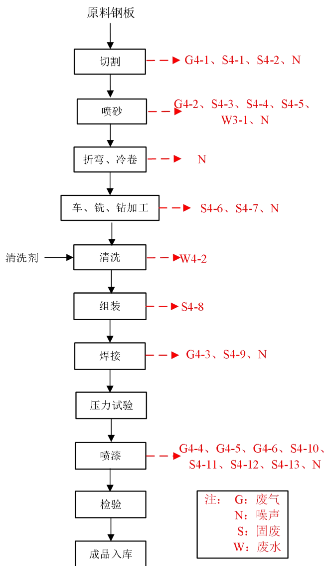
图 3-5 压力容器生产工艺流程图
