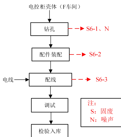
图 3-7 电控柜组装生产工艺流程图
