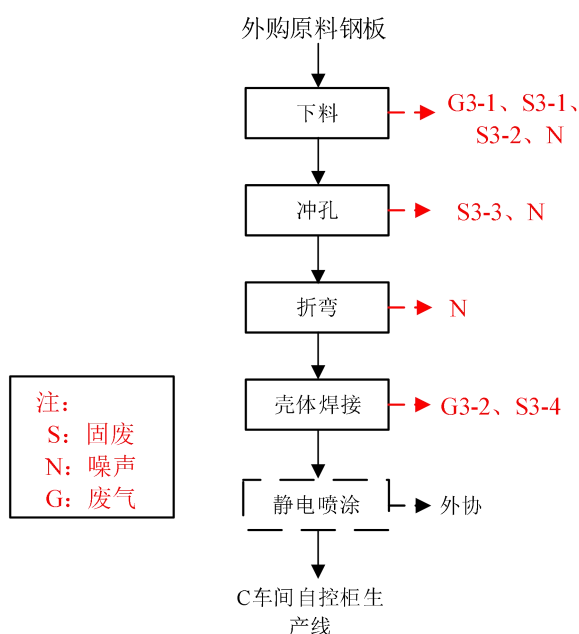
图 3-4 电控柜壳体生产工艺流程图
