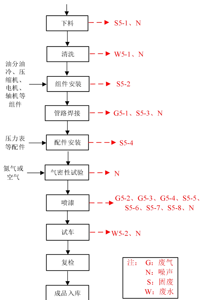
图 3-6 机组生产工艺流程图
